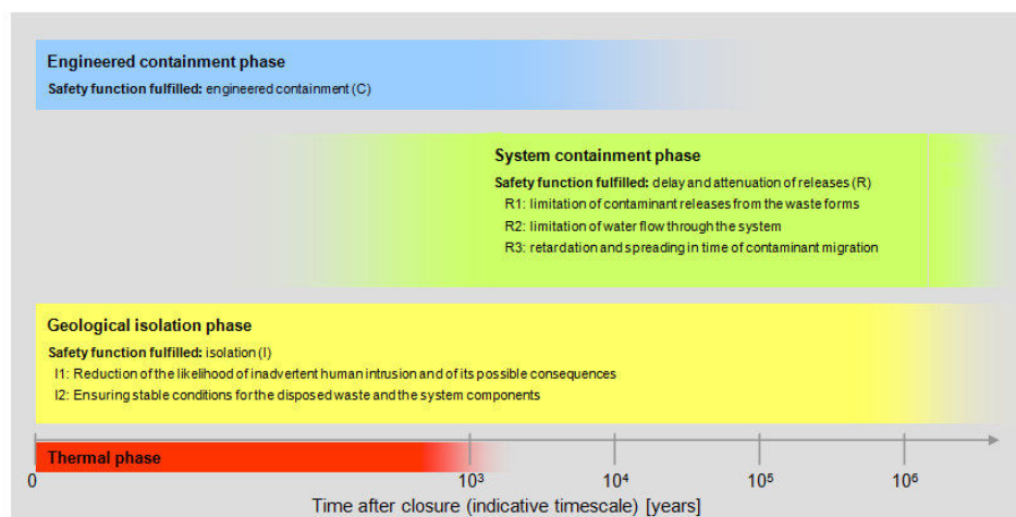
Figure 1 : Les fonctions de sûreté assurées sur le long terme par les composants du système de stockage développé par l'ONDRAF [8].
